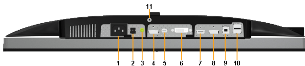
Vue de dessous sans le socle du moniteur
