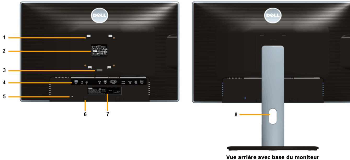
Vue arrière avec base du moniteur
